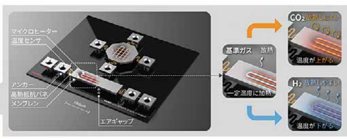
新技術での熱伝導型ガスセンサーの基盤の仕組みと動作原理:東芝のウェブサイトより
