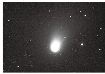
倉敷のアマチュア天文家が2023年1月に撮影した「ZTF 彗星」。これは2月に地球に約4200万キロの距離まで接近した。
