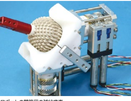
人型ロボットの関節用の球状歯車
