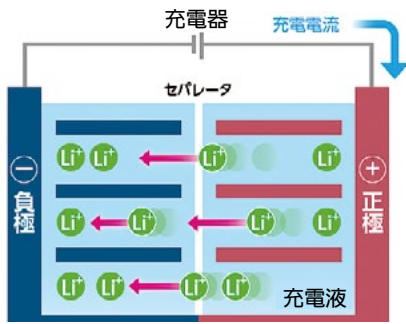
液体電解質の電池で、充電時にエネルギーを貯める時の様子。東芝 (株) のウェブサイトより 1. 充電器で電流を流す。2. 正極側にあるリチウムイオンが電解液を通過して負極側に移動。3. 正極と負極の間に電位差が生じて電池が充電される。
