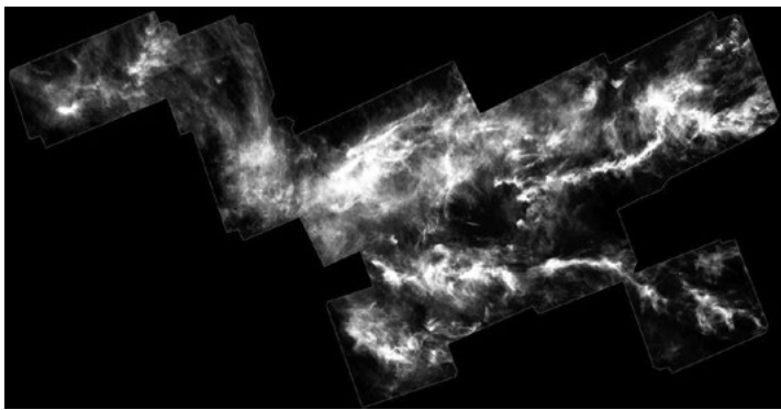
ハーシェル宇宙望遠鏡から見たおうし座分子雲のモザイク写真 画像出典: https://en.wikipedia.org/wiki/Taurus_Molecular_Cloud
